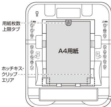
<トップカバー内部(上から見た図)>
