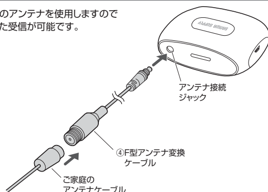
ご家庭のアンテナケーブル
