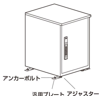
汎用プレート アジャスター
