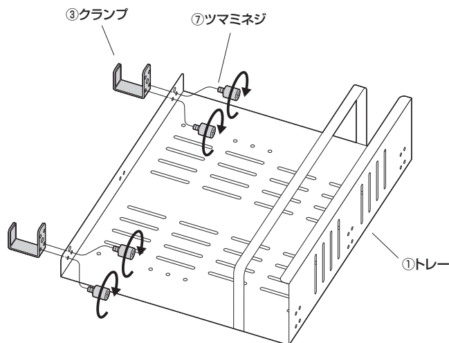
③クランプ
