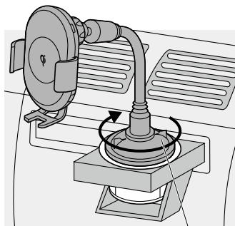
固定ノブ
