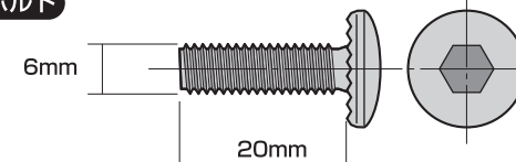
⑥ボルトA×4本 [M6×20]
