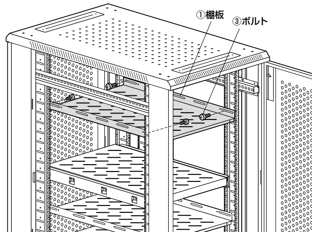
③ボルト (M6×12mm)
