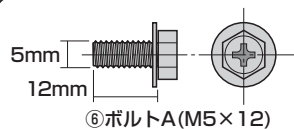
⑥ボルトA(M5×12)
