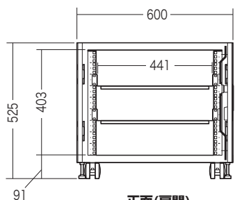
正面(扉開)
