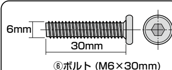
⑥ボルト (M6×30mm)
