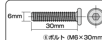
⑥ボルト (M6×30mm)
