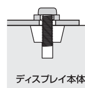
取付け穴断面図
