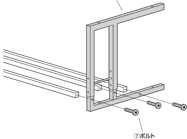
②サイドフレーム
