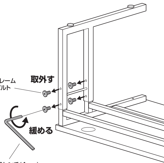
⑧六角レンチ(4mm)
