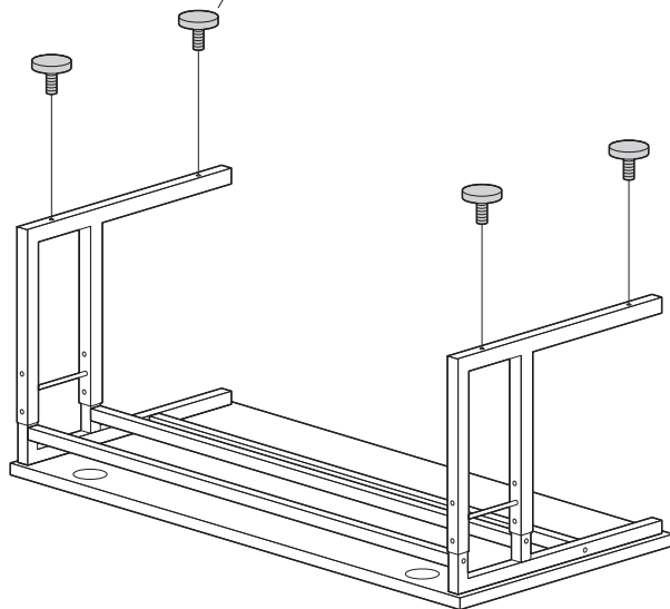
⑥アジャスター
