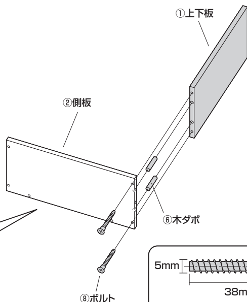
⑧ボルト
