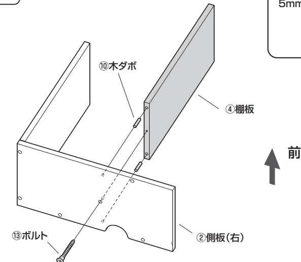
⑬ボルト(5×38mm)
