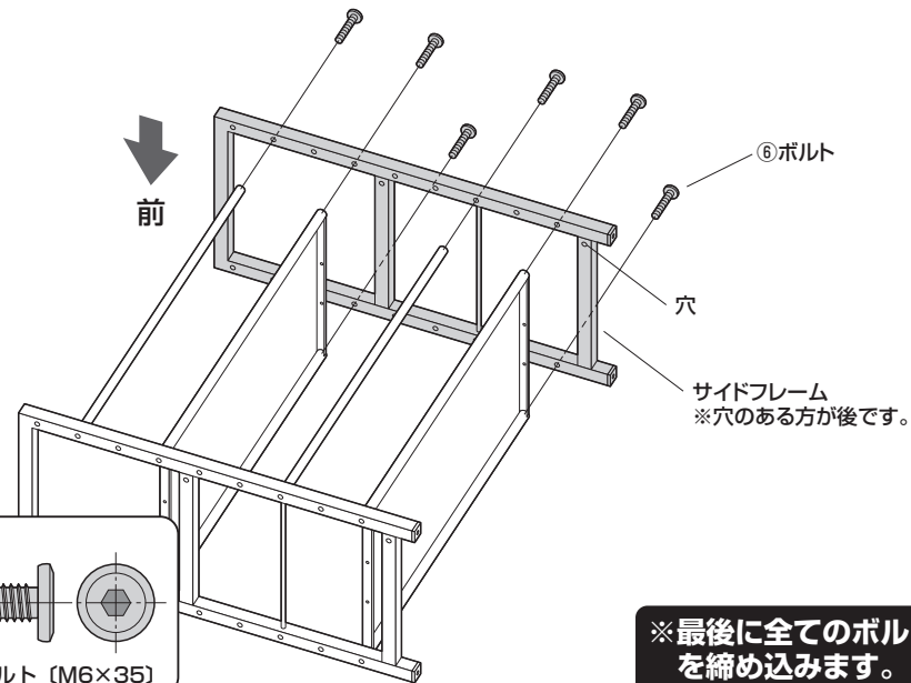
⑥ボルト (M6×35)
