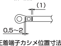
圧着端子カシメ位置寸法
