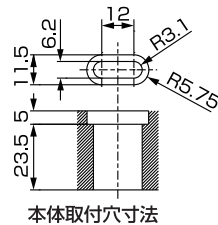
本体取付寸法
