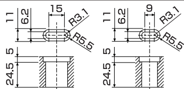
本体取付穴寸法
