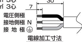
電線加工寸法
