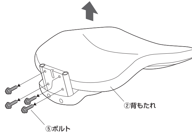
⑤ボルト
