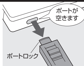
④取付け器具をポートロック と一緒に引き抜いてくだ さい。
