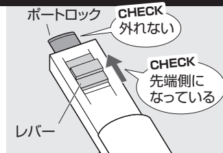
②レバーが先端側になっていて ポートロックが外れないこと を確認してください。
