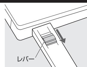
④レバーを手前にスライド し、ロックを解除してくだ さい。
