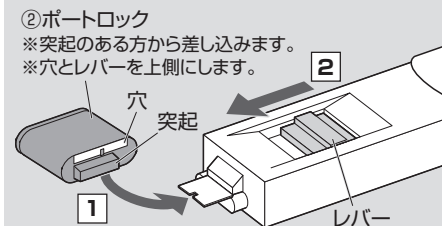
レバーを手前にした状態で、ポートロックを上図の向きで取付け器具の先端に取付け、レバーを先端側にスライドしてロックしてください。
