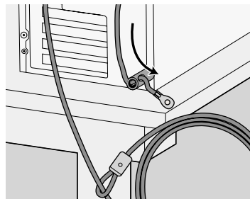
ワイヤーの片方を取付けたスチール製ブラケットに通します。
