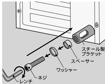
3種類あるネジから最適なものを選び、ワッシャー・スペーサーを間に入れてスチール製ブラケットに差し込み、レンチでしっかりと締めます
