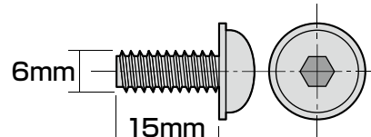
⑩ボルトA (M6×15mm)×20本
