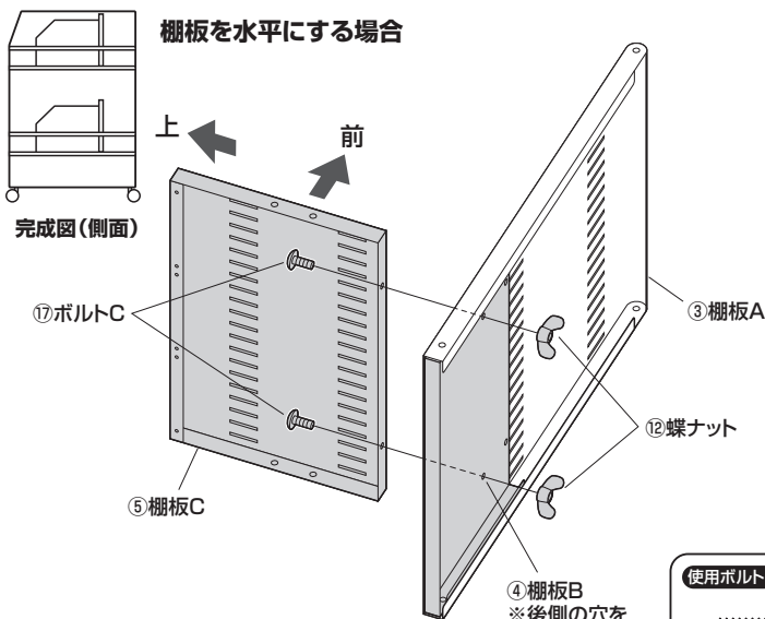
完成図(側面)
