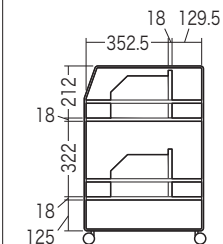
側面図A
