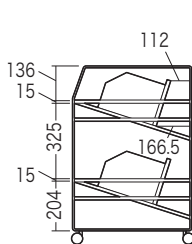
側面図B
