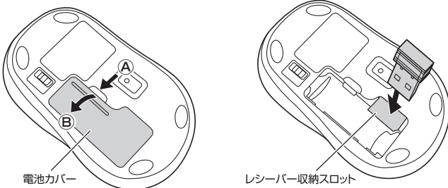
電池カバー
