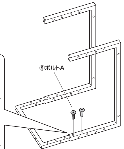
⑨ボルトA (M6×12mm)
