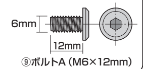
⑨ボルトA (M6×12mm)
