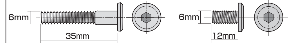
④ボルトA×12本(M6×35mm)
