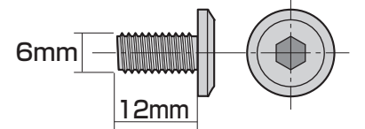
④ボルトB×4本(6×12)
