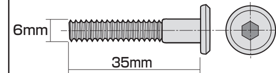
③ボルトA×4本(6×35)
