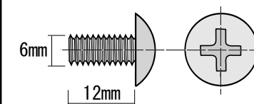
③スクリュー [M6×12] ×4本
