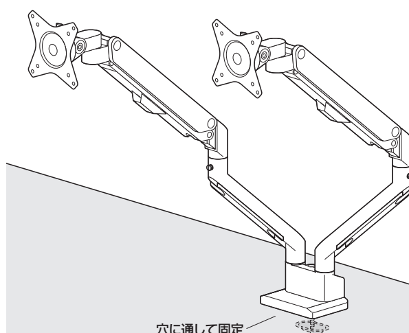
⑥ボルトA(M8×130mm)×1本
