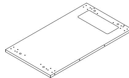
㉑底板 × 1
