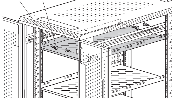
①棚板 ③ボルト
