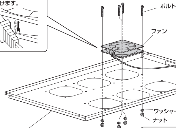
⑫ファン用ブラケット
