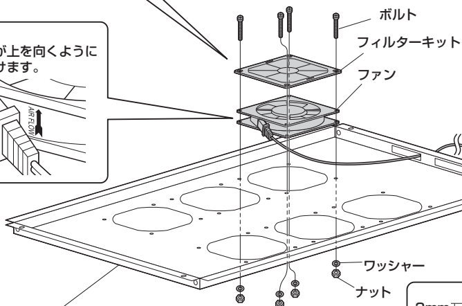
⑫ファン用ブラケット
