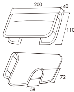
カバー寸法図
