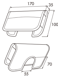
カバー寸法図
