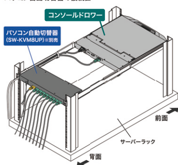
パソコン自動切替器の接続図
