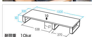
幅530mmまでのキーボードが収納できる。フレーム底面には滑り止め付き。
