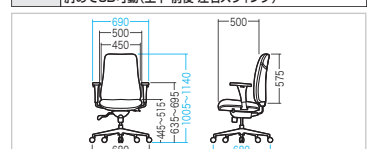
肘あては3方向へ調整可能。肌触りの優しいPU製。
